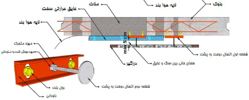
ب- نمونه ای از اجرای دوخت به پشت نمای سنگی به دیوار در محل مسلح سازی دیوار شکل پ ۶-۳۰- نمونه‌هایی از اجرای دوخت به پشت نمای سنگی به دیوار و جزئیات اجرایی آن
