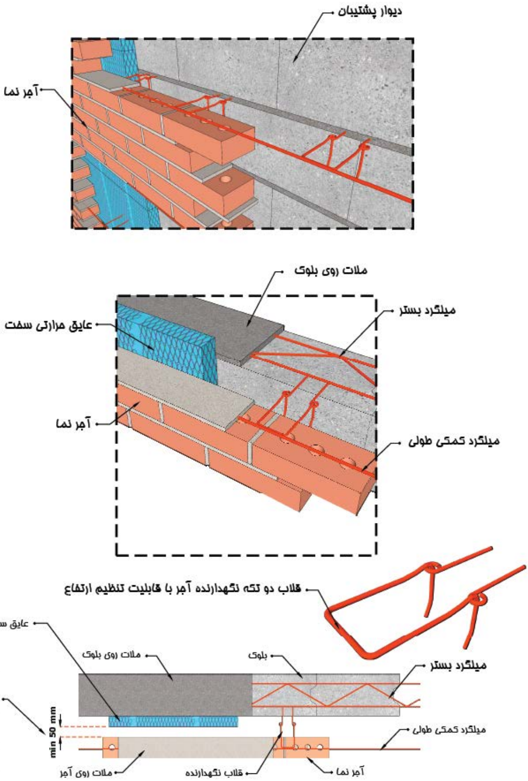
شکل پ-۲۸-۶- نحوه مهار نمای آجری به دیوار پشت
